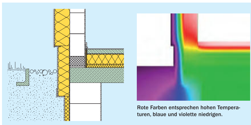
Bild 7 Hochwertige Details als Grundlage für hohe Energieeffizienz
