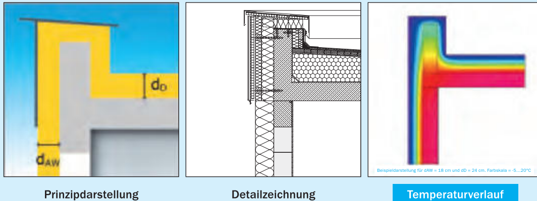
Bild 17 Wärmebrückendetail Traufe/Attika: Beim Übergang zum Dach kann sowohl beim Schrägdach ein Übergang ohne relevante Verringerung der Dämmdicke erreicht werden als auch bei Ausführung einer Attika beim Flachdach, bei der negative Wärmebrücken Standard sein sollten
