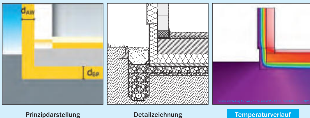
Bild 19 Wärmebrückendetail Sockel nicht unterkellert: Die Dämmung der Außenwand geht vollflächig in die Dämmung unterhalb der Bodenplatte über, wodurch die Wärmeverluste im Sockelbereich minimiert werden können
