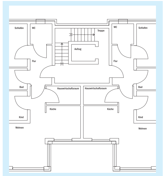
Bild 4 Aufzugsschacht zentral im Treppenraum ist wirtschaftlich mit KS-Mauerwerk ausführbar
