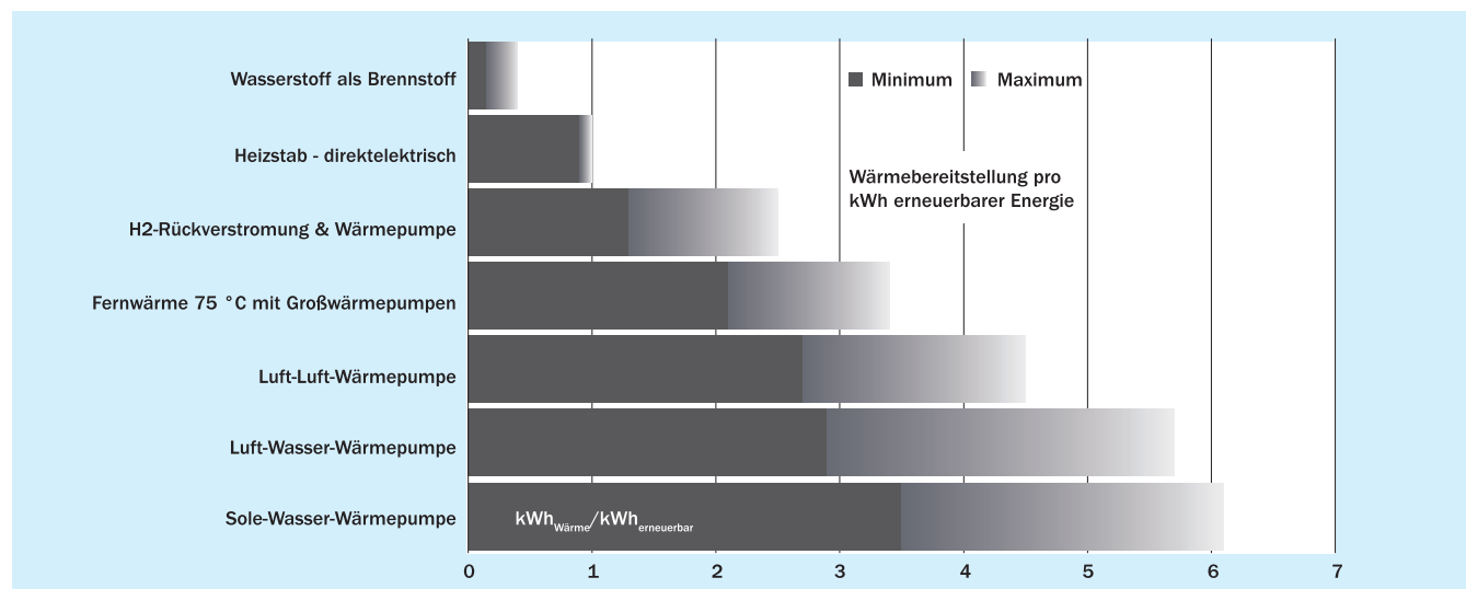
Bild 24 Effizienz von Heizsystemen im Vergleich: Anteil der nutzbaren Wärme pro kWh erneuerbaren Stroms
