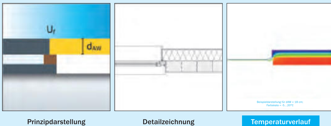
Bild 18 Wärmebrückendetail Fensteranschluss: Fenster werden so montiert, dass der Rahmen möglichst weitgehend von Dämmung umfasst wird. Dadurch ergeben sich sehr geringe Einbauwärmeverluste im Bereich von 0,01 W/(mK)
