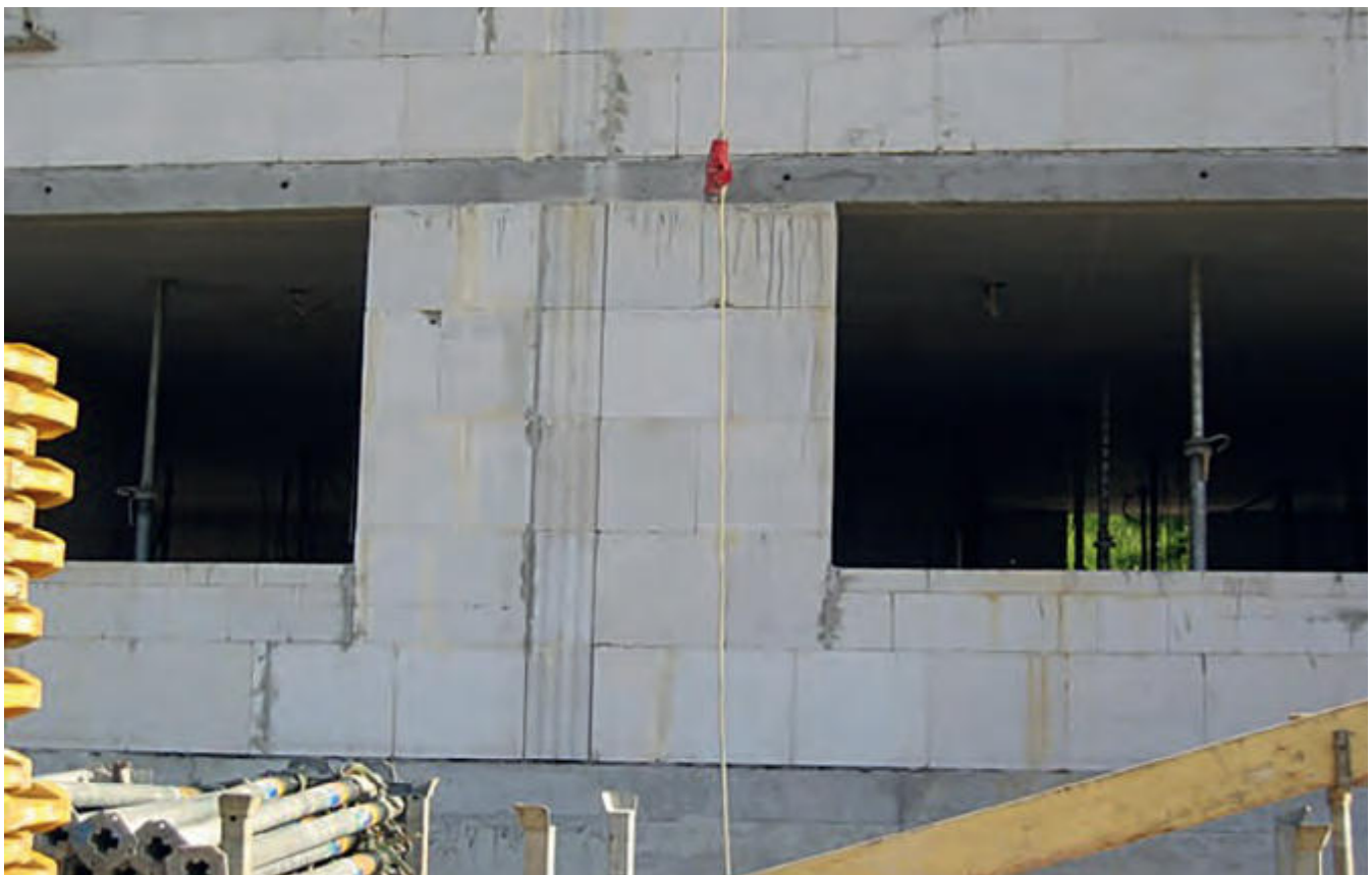
Bild 8 Durchgehende Wohnungstrennwand als Beispiel für eine optimierte schalltechnische Planung
