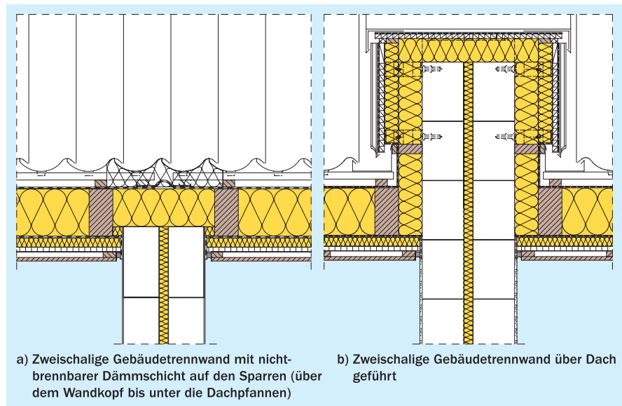
Bild 7 Gebäudeabschlusswand aus KS-Mauerwerk im Dachbereich
