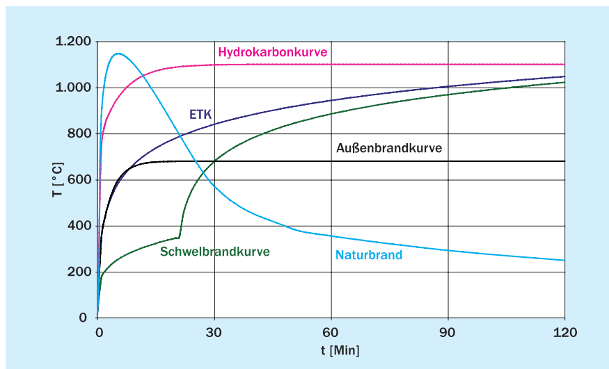
Bild 3 Temperaturprüfkurven – Brandeinwirkungen
