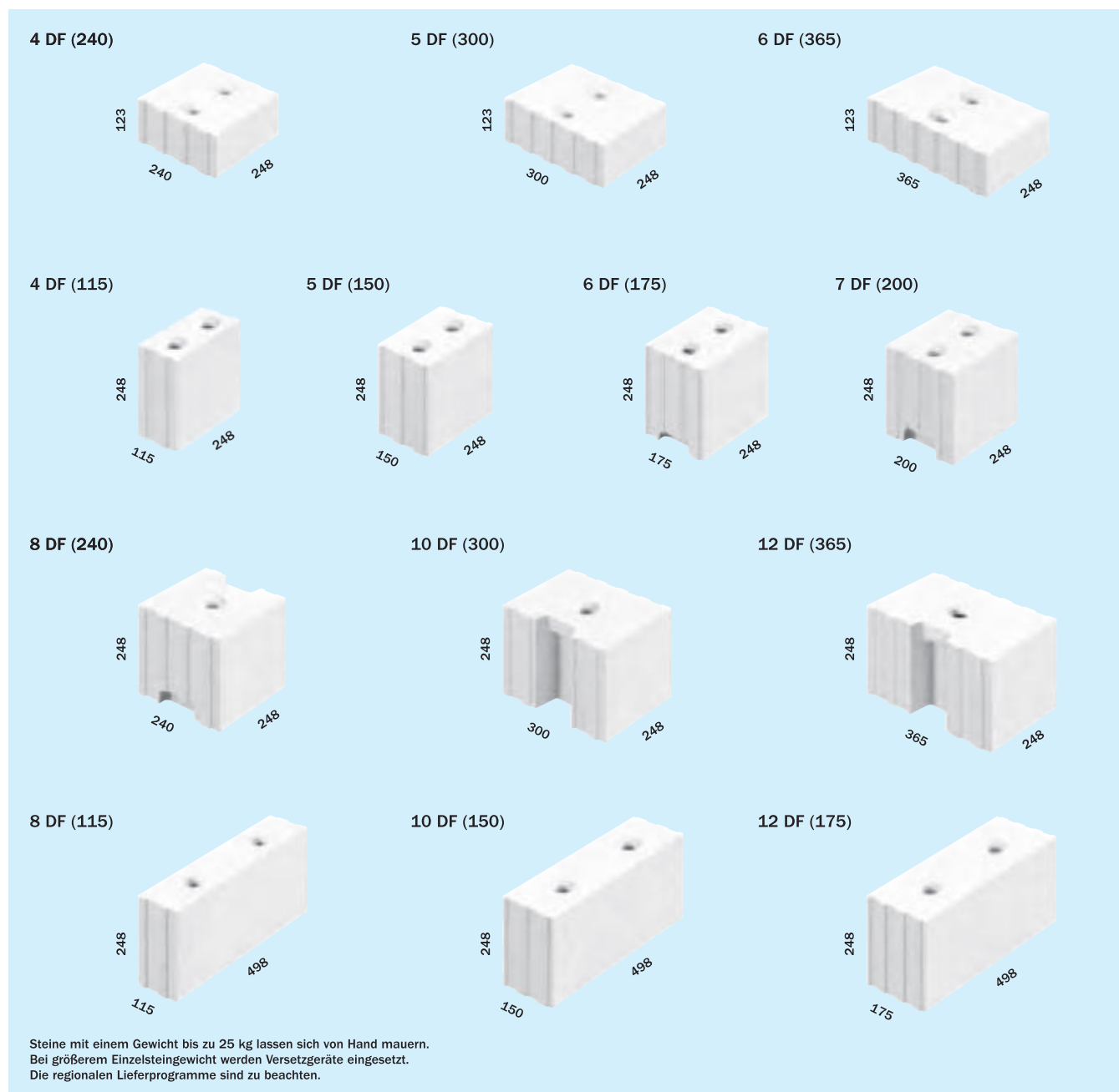
Bild 9 Beispiele von KS -R-Plansteinen ( h = 123 \text{ mm} bzw. 248 \text{ mm} ) zur Verarbeitung mit Dünnbettmörtel
