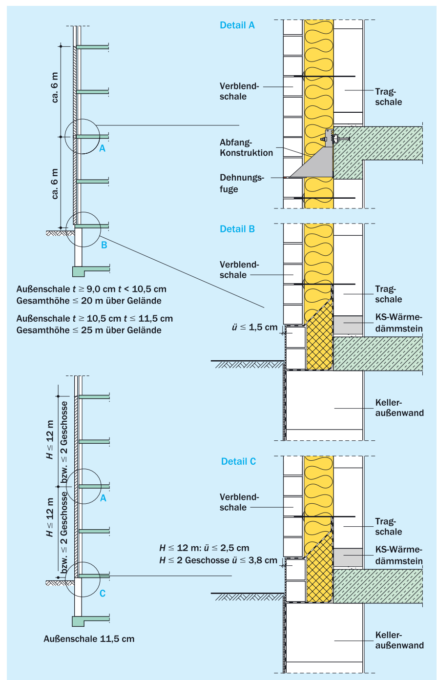
Bild 8 Randbedingungen zur Ausführung von zweischaligen Außenwänden nach DIN EN 1996-2/NA [3]
