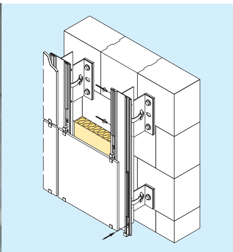
Bild 35 Vorgehängte hinterlüftete Fassaden mit Aluminium-Unterkonstruktion
