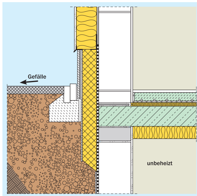
Bild 23 Verzicht auf zusätzlichen Feuchteschutz, da der WDVS-Sockel nicht verputzt, sondern mit einer Bekleidung überdeckt ist
