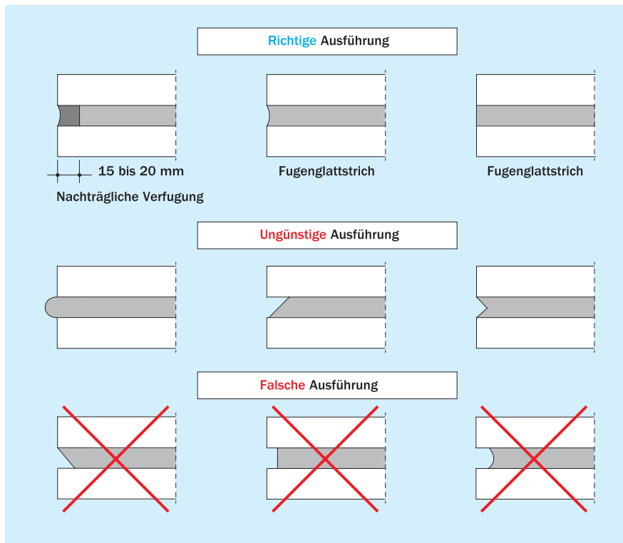
Bild 9 Ausführung von Mörtelfugen bei Verblendschalen
