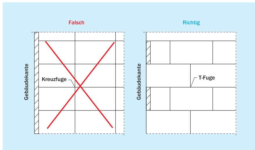
Bild 31 Verlegung von WDVS-Dämmplatten im Verband im Regelquerschnitt
