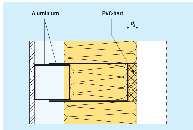
Bild 39 Reduzierung der Wärmebrücke am Wandhalter
