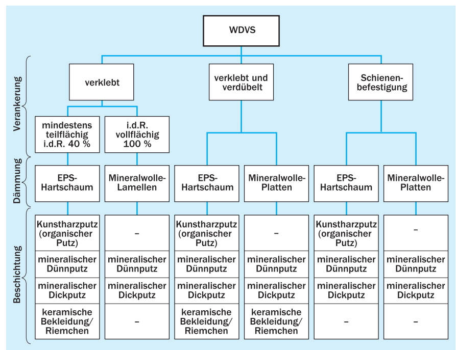
Bild 19 Übersicht der marktüblichen Wärmedämmverbundsysteme
