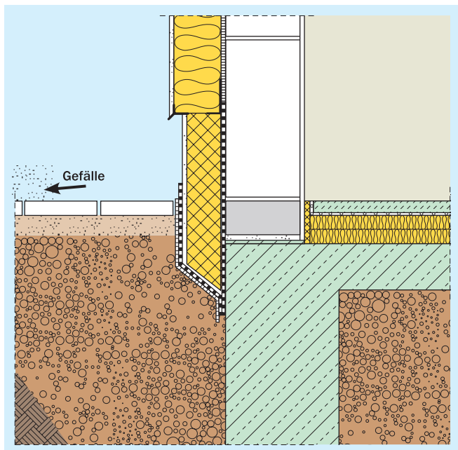
Bild 22 Zusätzlicher Feuchteschutz des verputzten WDVS-Sockels
