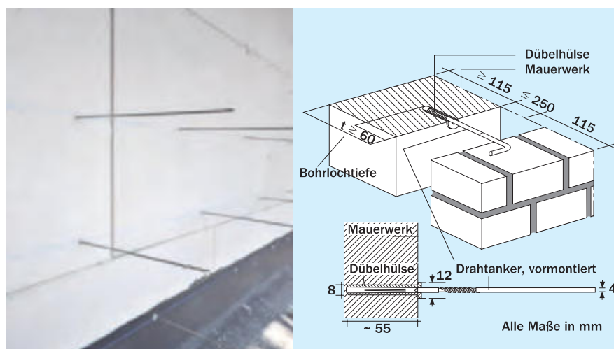
Bild 7 Dübelanker
