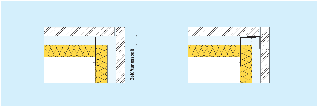
Bild 37 Vertikale Windsperren an Gebäudekanten
