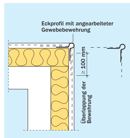
Bild 30 Kantenprofil
