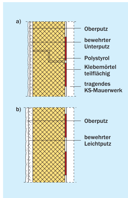
Bild 20 Teilflächig verklebtes WDVS mit EPS-Dämmplatten
