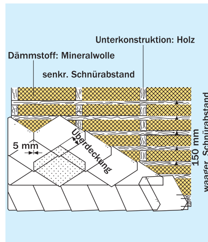
Bild 36 Vorgehängte hinterlüftete Fassaden mit Holz-Unterkonstruktion
