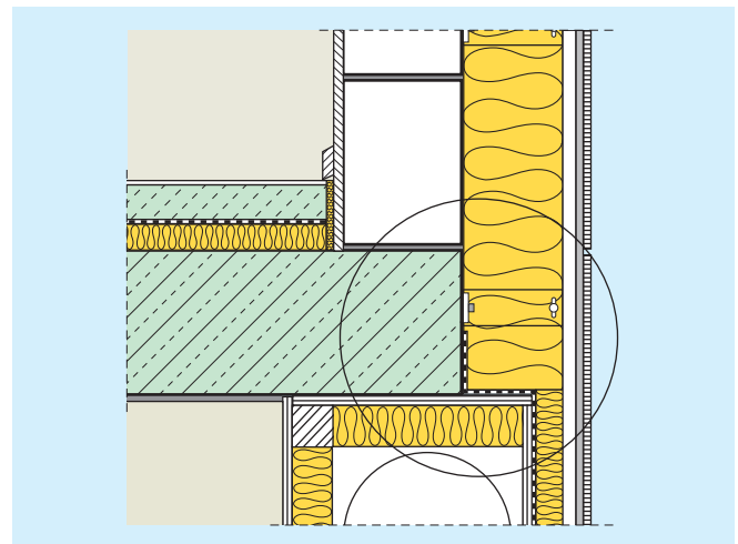
Bild 40 Fußpunktabdichtung bei vorgehängten hinterlüfteten Bekleidungen (aus FHV 21 [44])
