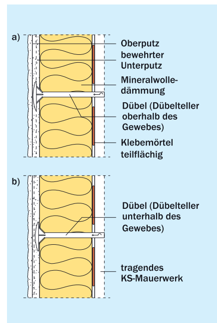
Bild 21 Teilflächig verklebtes und verdübeltes WDVS mit Mineralwolle-Dämmplatten
