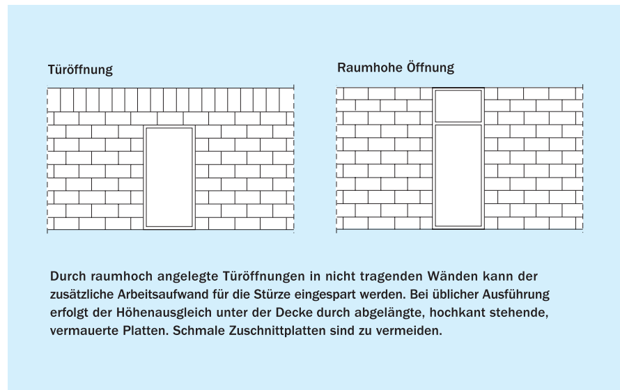
Bild 9 Türöffnungen
