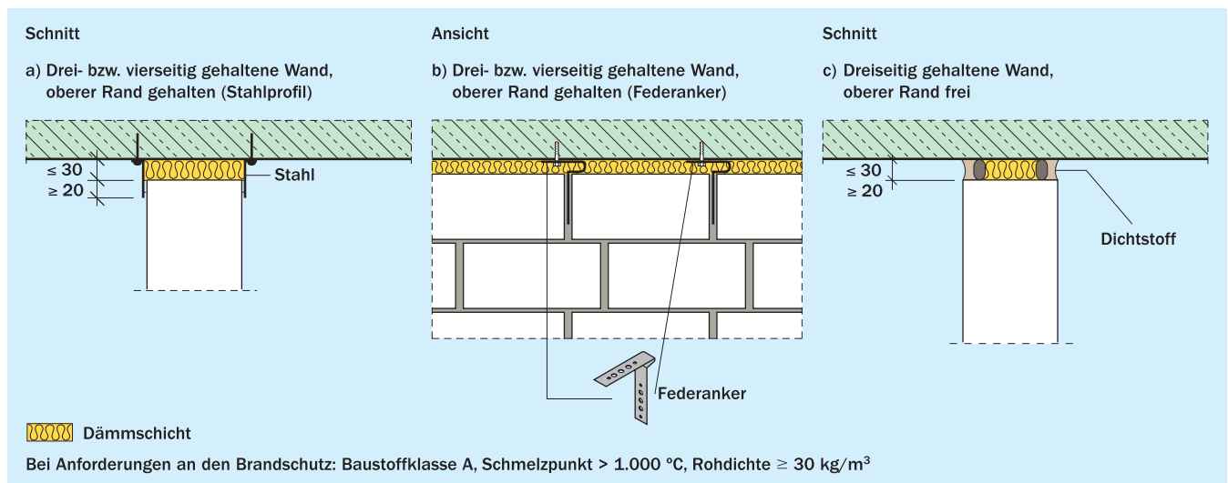
Bild 8 Deckenanschlüsse (gleitend)
