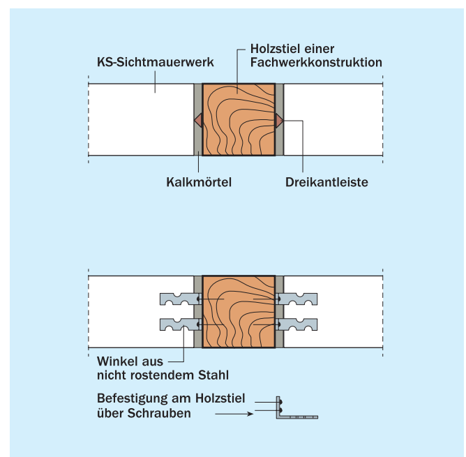
Bild 2 Wandanschluss von KS-Sichtmauerwerk an eine Holzfachwerkkonstruktion
