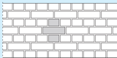
Kreuzverband
