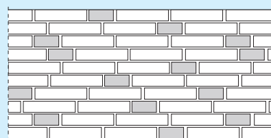
Wilder Verband
