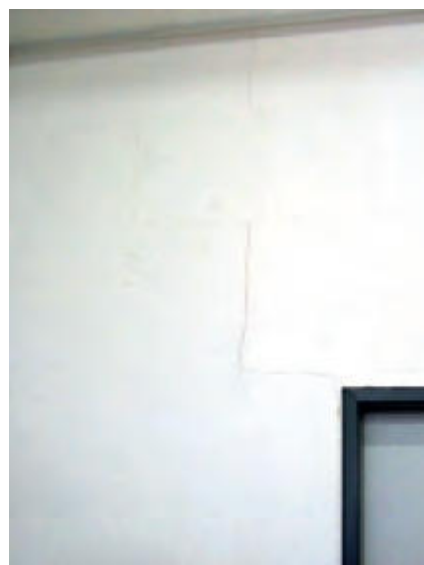
Bild 24 Rissbildung in nicht tragender Trennwand infolge Durchbiegung der unteren Geschossdecke
