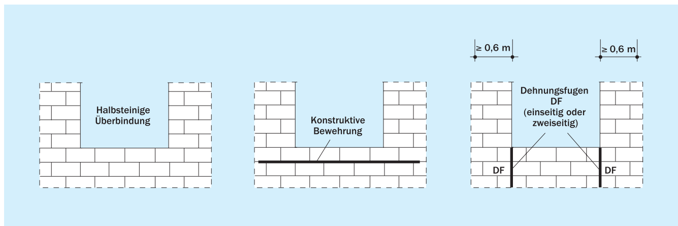
Bild 41 Brüstungsbereiche von Verblendschalen
