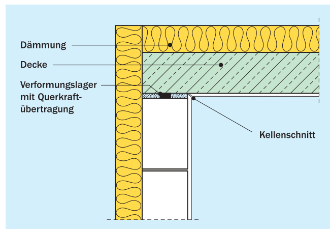
Bild 31 Konstruktive Maßnahmen zur Zentrierung der Deckenauf-lagerkraft am Beispiel der Außenwand unter einer Dach-decke – Verformungslager mit Zentrierstreifen zwischen Wand und Decke
