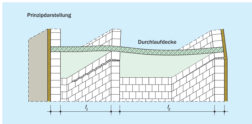
Bild 28 Rissbildung infolge großer Deckendurchbiegung
