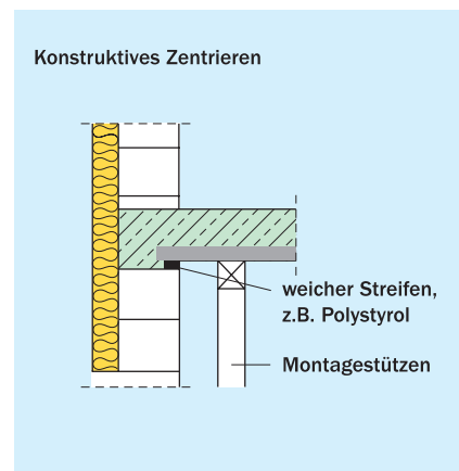
Bild 29 Einlage weicher Streifen zur Lastzentrierung
