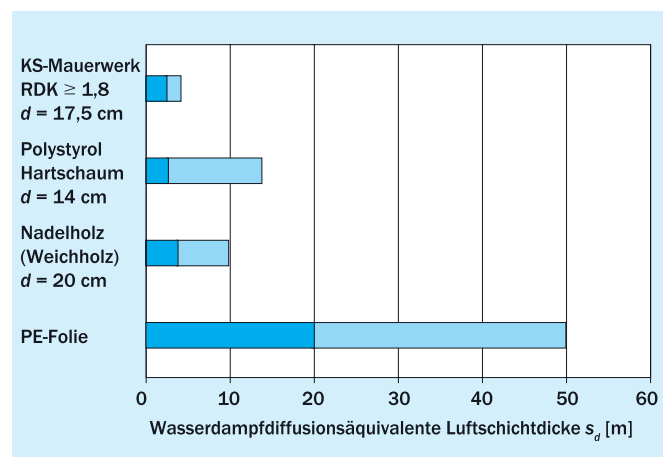
Bild 19 Wasserdampfdiffusionsäquivalente Luftschichtdicke s_d ausgewählter Baustoffe, jeweils für den Kleinst- und den Größt-wert des \mu -Werts nach DIN 4108-4 bzw. nach DIN EN 12524
