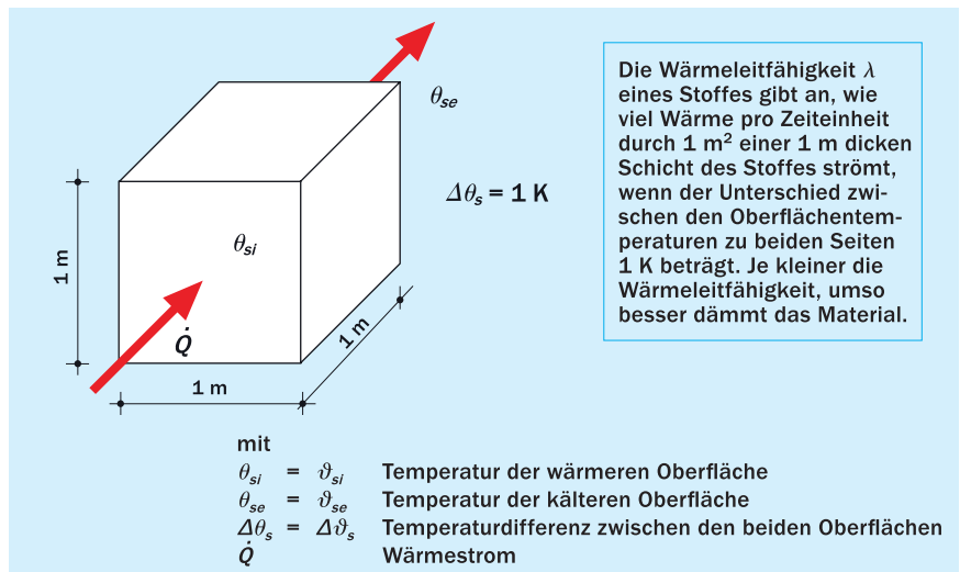
Bild 6 Wärmeleitfähigkeit
