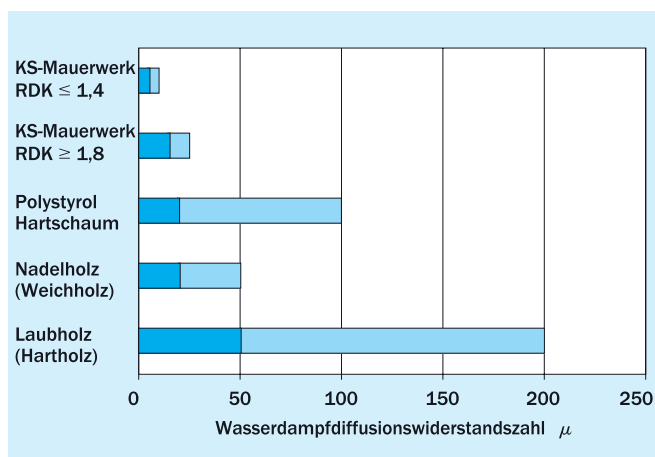
Bild 18 Wasserdampfdiffusionswiderstandszahlen ausgewählter Materialien, angegeben sind jeweils Kleinst- und Größt-wert nach DIN 4108-4 bzw. nach DIN EN 12524
