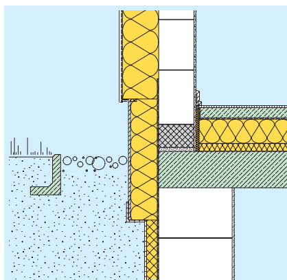
Bild 14 Konstruktionszeichnung aus KS-Detaillenkatalog, Detail 2.2.3
