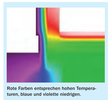
Bild 15 Temperaturverlauf am Anschlussdetail von Bild 14
